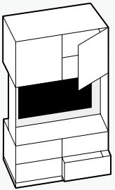
① 1200 TV장 너비(W) 1200(42" TV 권장) 깊이(D) 625
